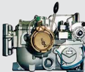
PRECIMA 800 • 800 l/min flexible plein et en flexible vide
